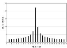
彰化地區控制雨量站：下水埔雨量分配圖(Hornner)
