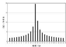
彰化地區控制雨量站：臺西雨量分配圖(Hornner)
